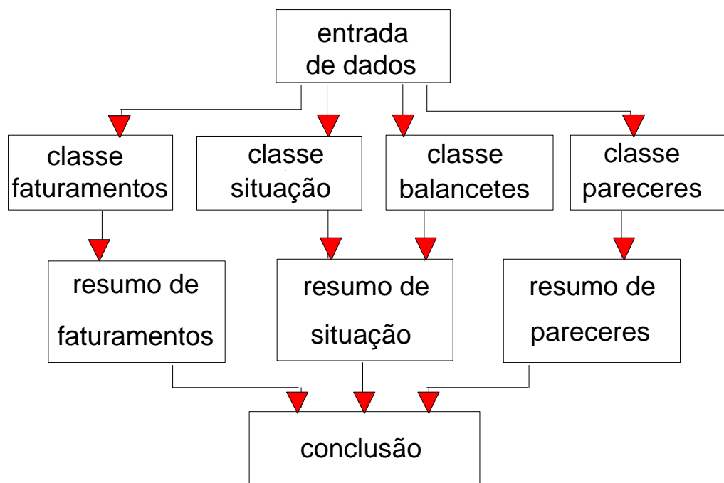
Figura 3.1 - Esquema básico do encadeamento para frente
