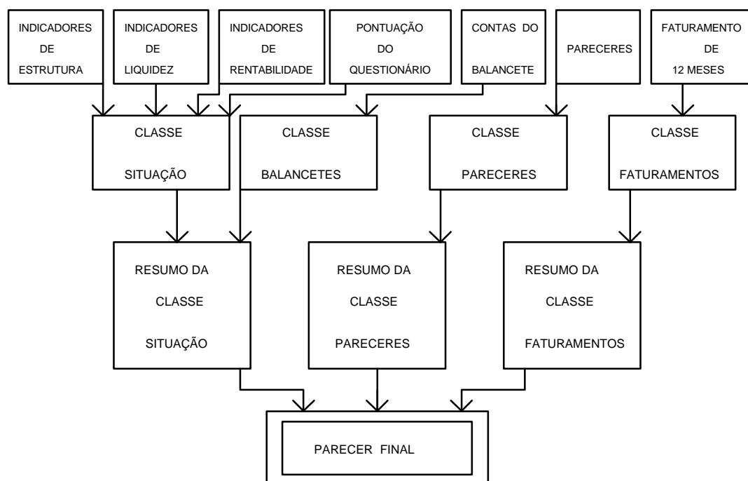
Figura 3.4 - O Raciocínio do SENACRE
